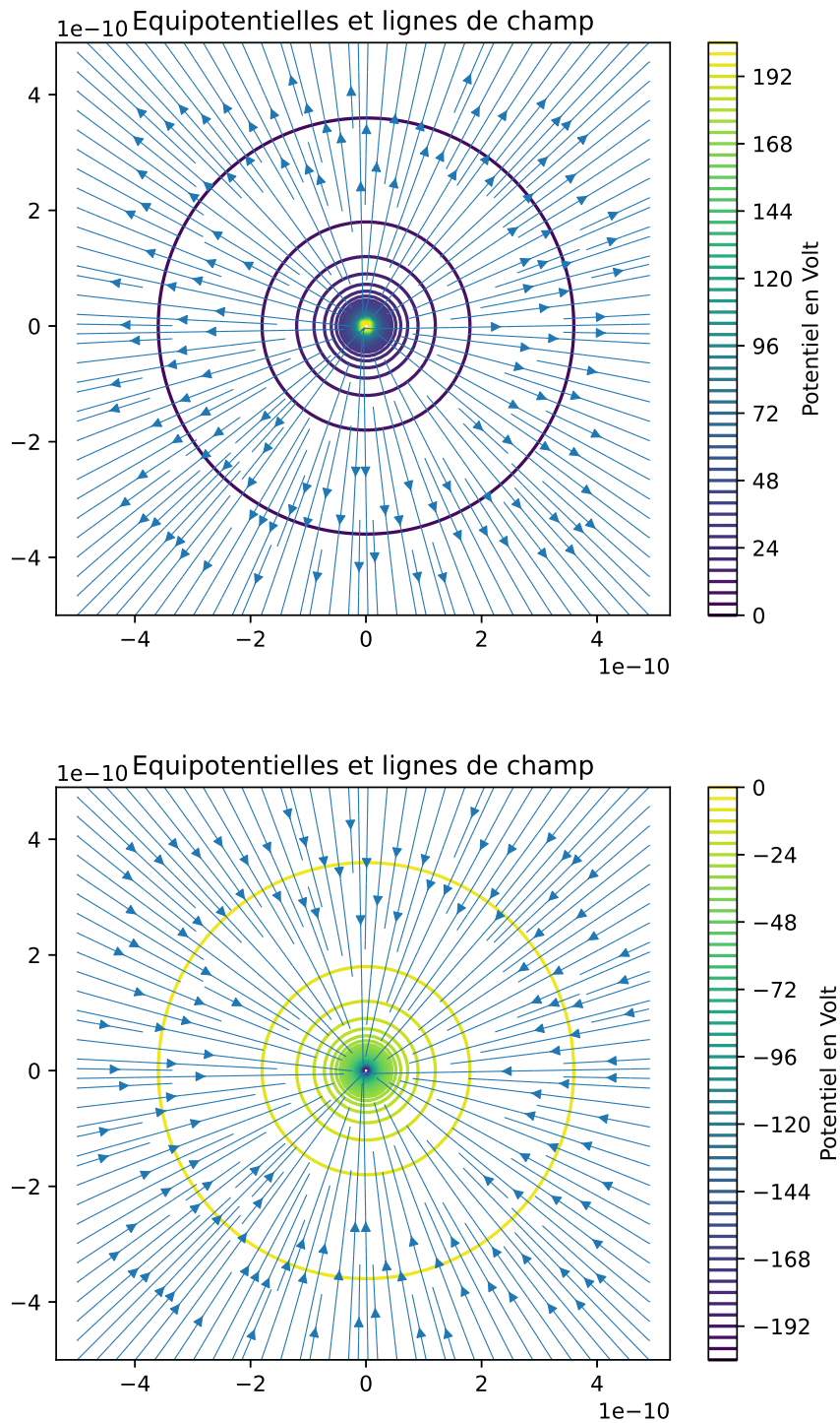
FIGURE 2 – Proton ou électron placé à l'origine du repère
