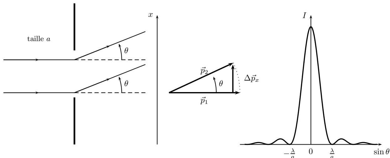
FIGURE 5 – Diffraction de FRAUNHOFER par une fente
